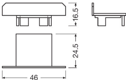
729013_FX-QMW-G1-EFGP-TU26H25W10
